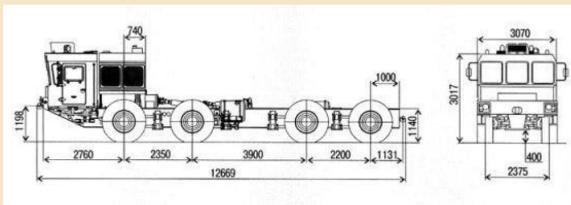
Рис. 2. Схема шасси МЗКТ-7930. Источник: Volatdefence.com
